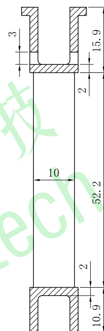
SECTION D-D
